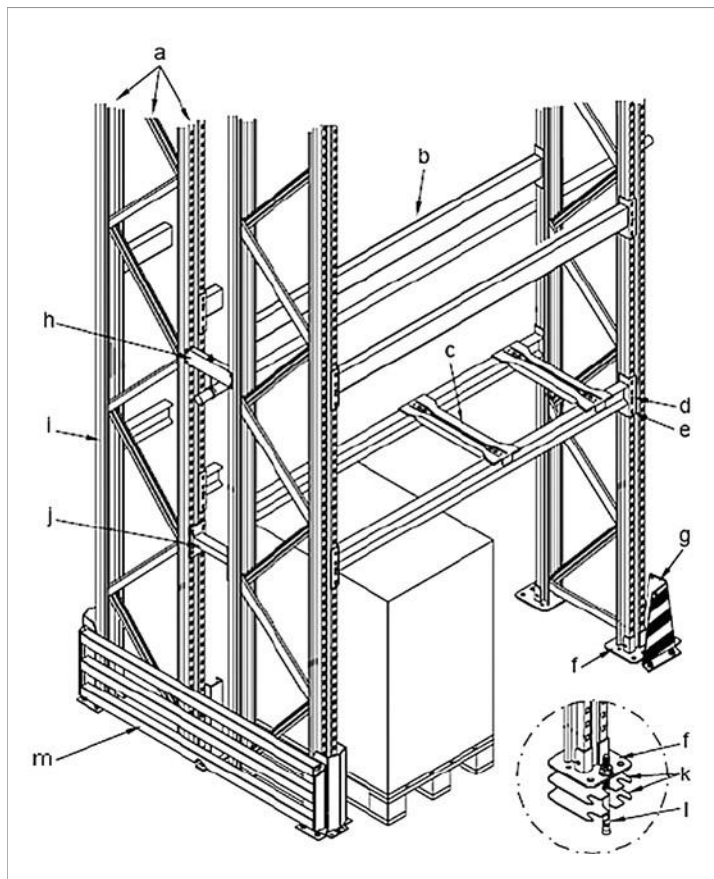
Fig. 7 - Scaffalatura portapallet. Componenti generali ed accessori. Legenda: a) spalla, b) corrente, c) elemento di ripartizione, d) connettore, e) spina antigancio, (b) ed orizzontale (a). f) piastra di base, g) paracolpi, h) supporto per sprinkler, i) montante, j) distanziale, k) piastra, l) spessoramento, l) tassello di ancoraggio, m) barriera di protezione.
